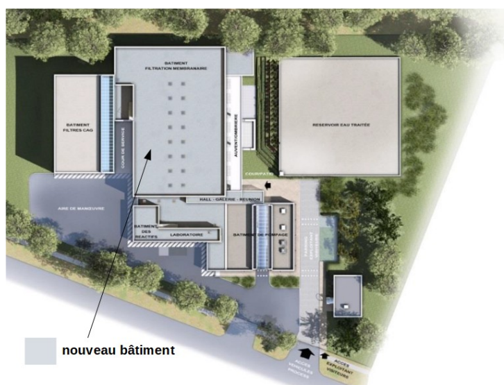
Illustration 2 : projet sur le site de l'usine (étude d'impact, p. 23 – modifié par MRAe)
