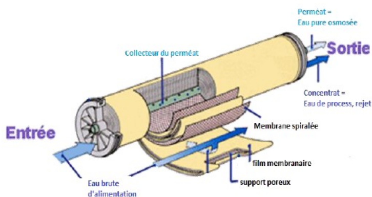
Illustration 3: filtration membranaire (étude d'impact, p. 18)
